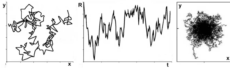
Рис. 1. Траектории броуновской частицы в однородной среде (система самоподобна и может быть охарактеризована показателем фрактала d_f ).
