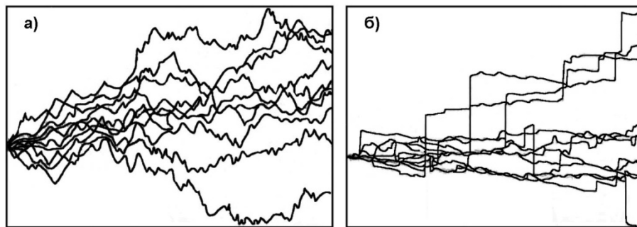
Рис. 2. Модели случайного блуждания: а – броуновская диффузия; б – процесс Леви.
